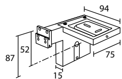
923828 Lato perno Carena Pivot side Carena Côté pivot Carena Träger Achseseite Carena Lado pivote Carena Strona czopa Carena
