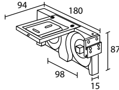
923469 Doppio C Double C Double C Doppelträger C Doble C Podwójny C
